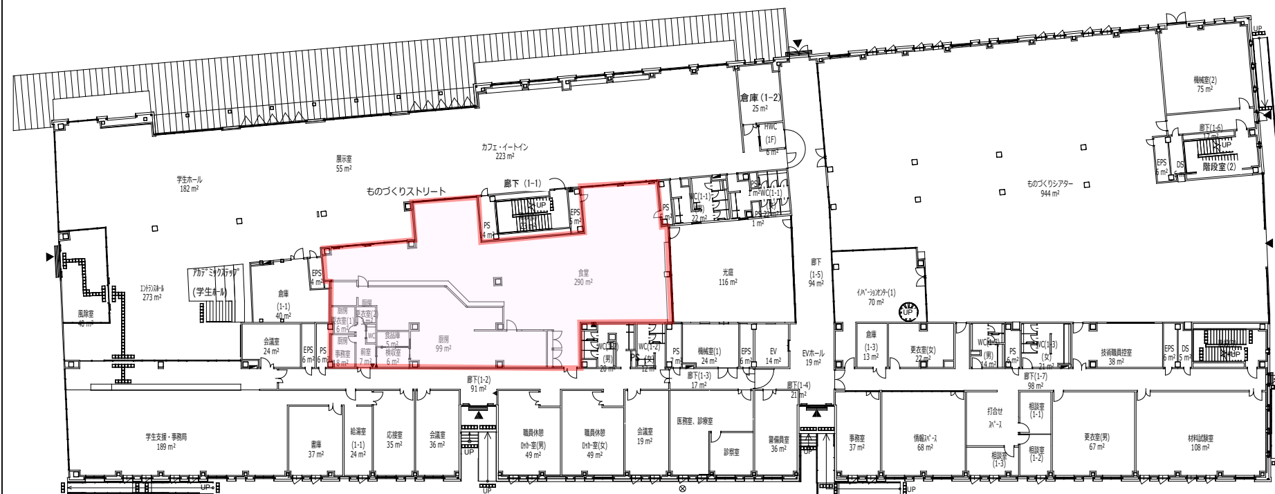
1階平面図
