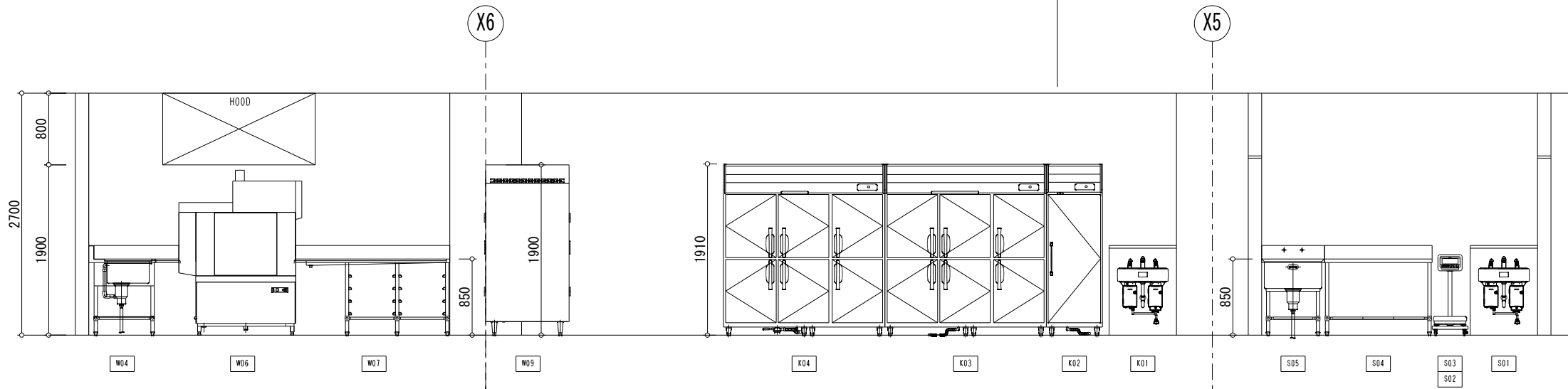
C方向展開図
