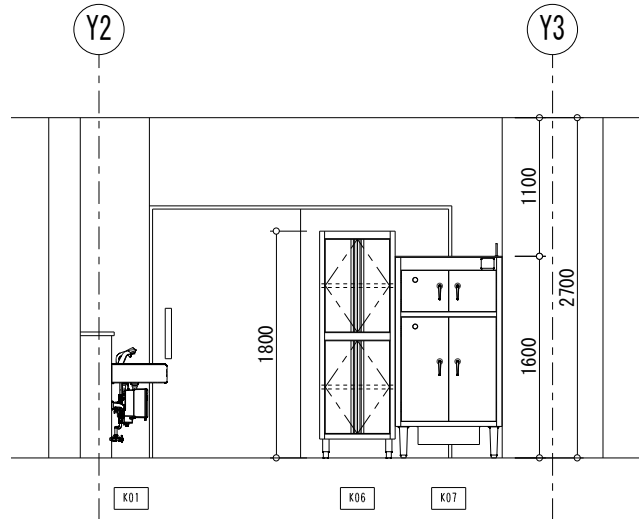
A方向展開図
