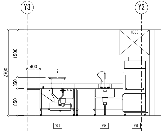
B方向展開図
