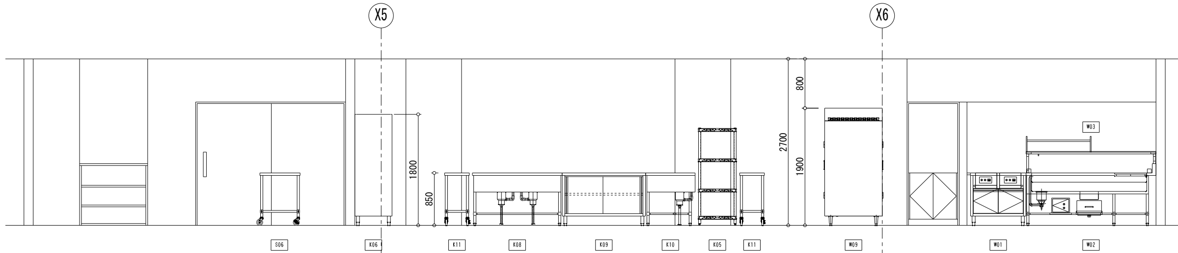
D方向展開図
